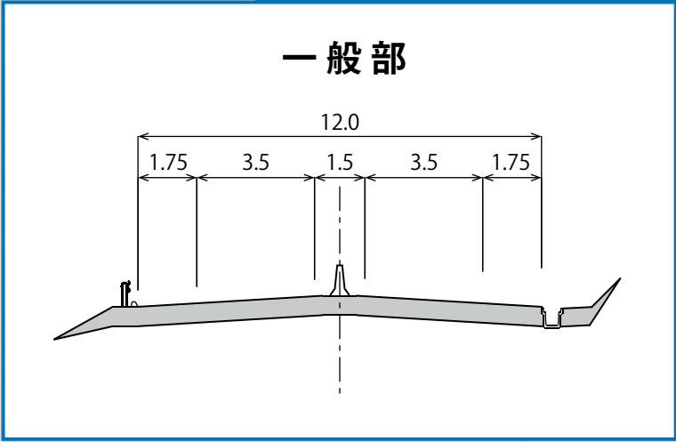
標準断面図 (単位:m)
