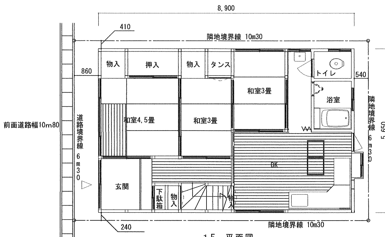
1 F 平面図
