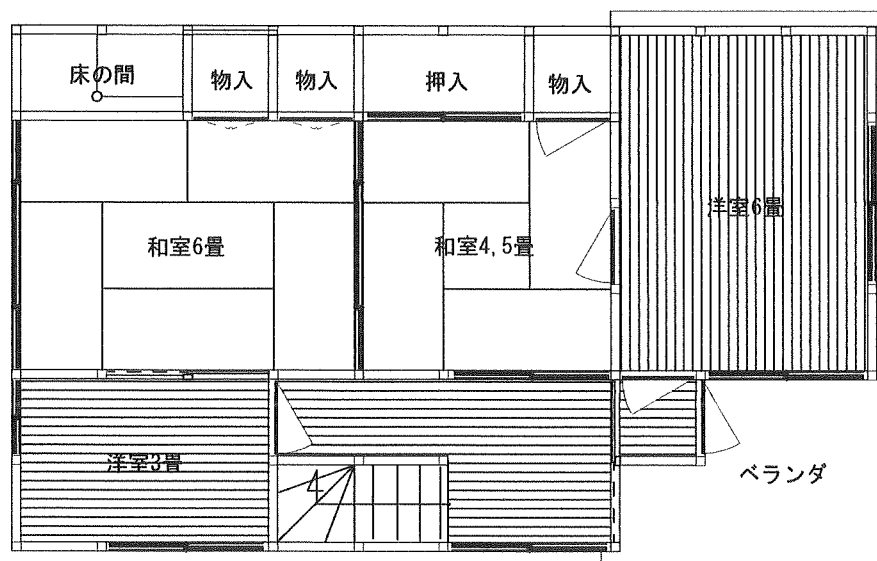
2 F 平面図
