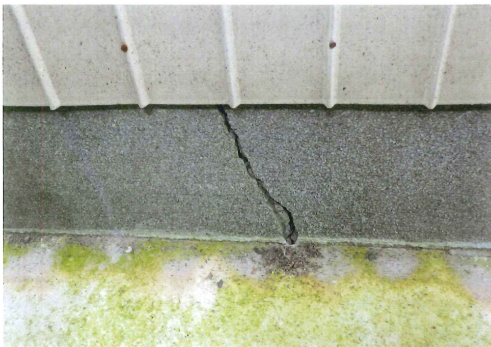
2-① 地盤の沈下による基礎の割れ。
