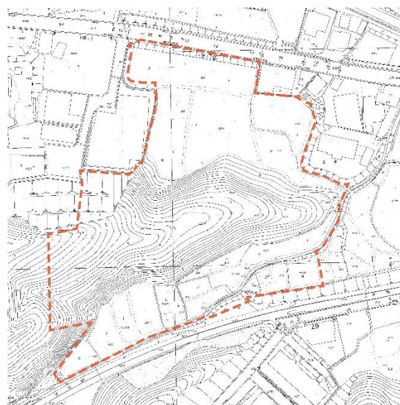
現況敷地図
