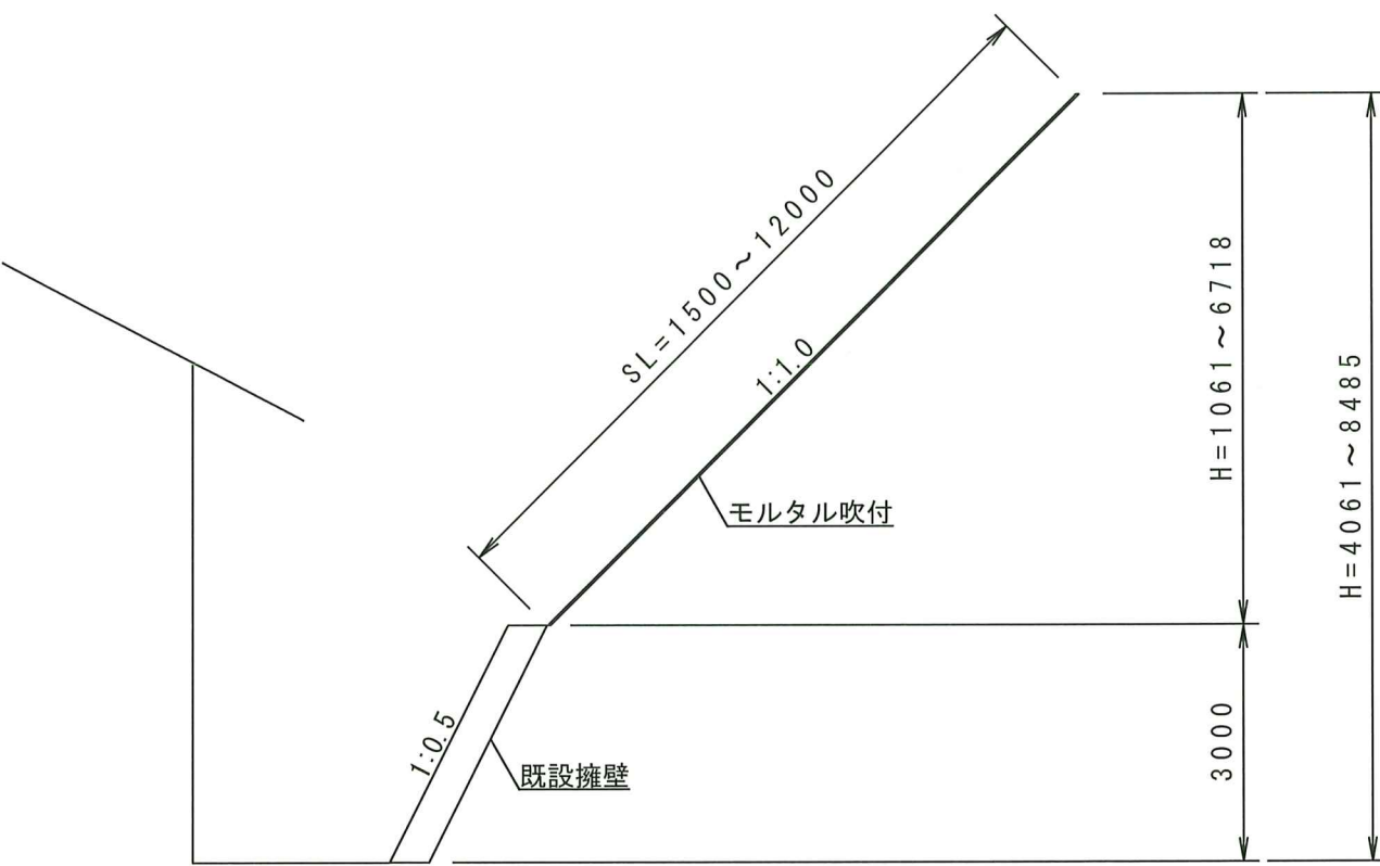
標準断面図 s=1/100
