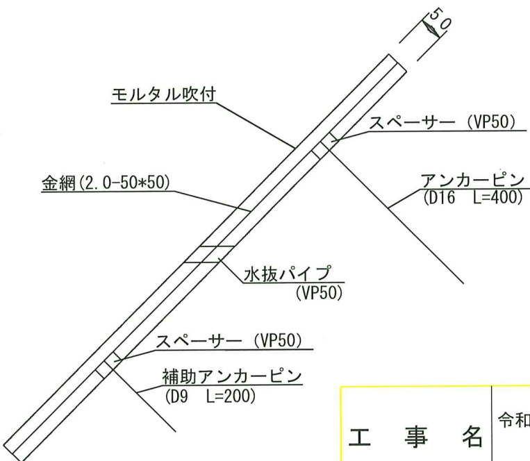
モルタル吹付詳細図 s=1/10
