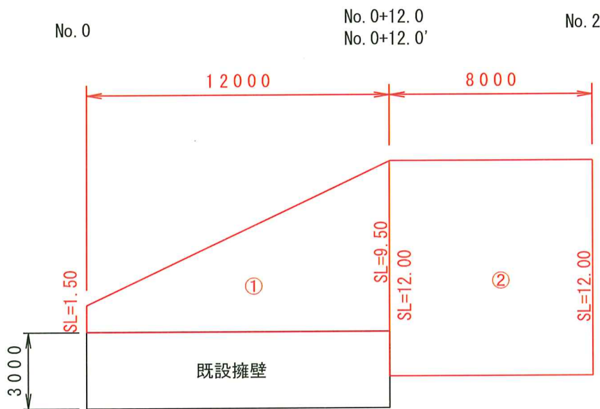
展開図 s=1/200
